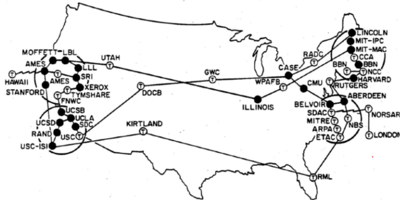
Slika 37 ARPANET 1970 godine
